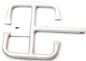
Referência 14.GA024C Dimensões 390x260x20 mm
