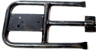
Referência 14.GA024D Dimensões 330x260x20 mm
